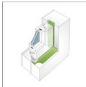
Overgang van TP650 illmod Trio naar illbruck TP651 illmod Trio S.
