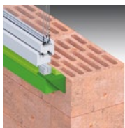
Sustav 2: 90 mm preklopa
