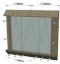
Bild 8: Sicherungsschrauben BLK-Tür 3-flg.
